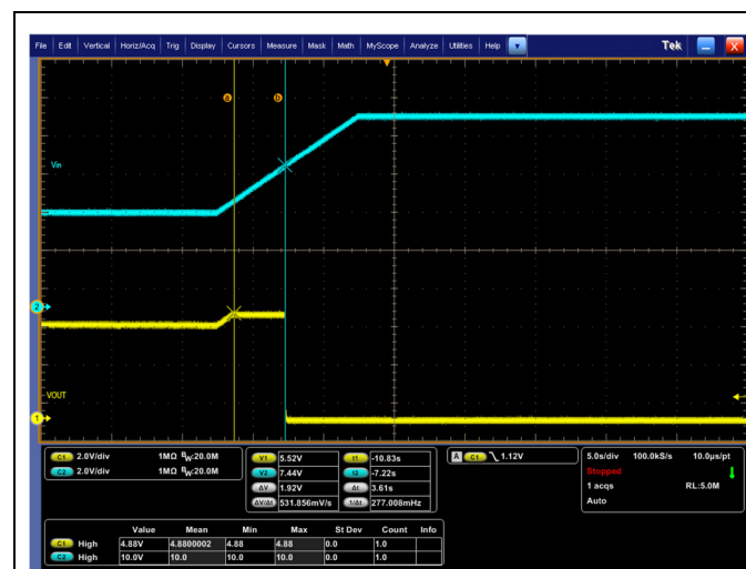
Fig. 1: Main_OVP
